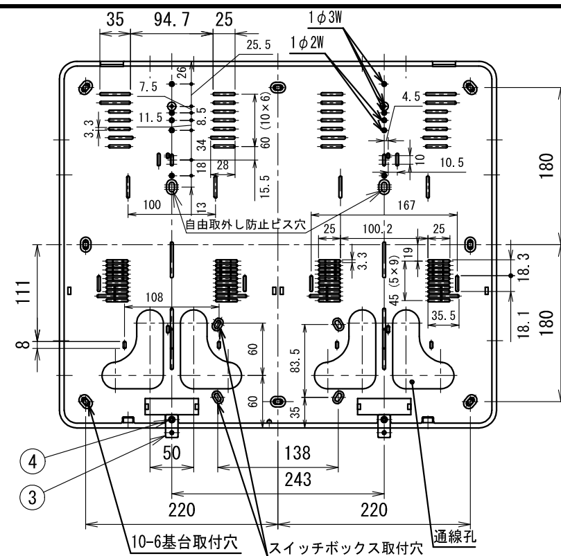
基台詳細図
